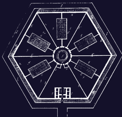
Pianta ed elevazione geometrica del gran Carcere centrale di AVELLINO in Principato Ultraiore.
